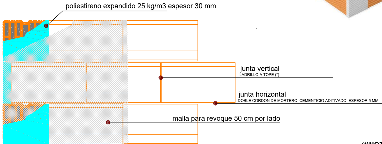
VISTA
